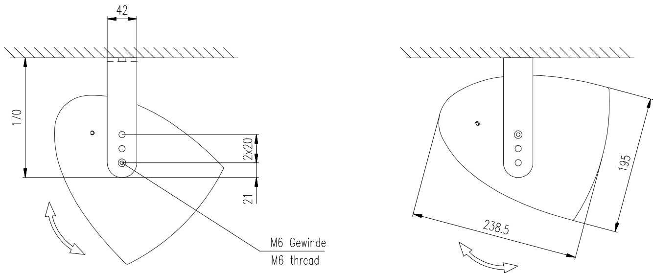
Seitenansicht / Side view
