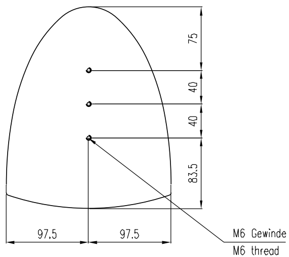
Bodensicht / Bottom view
