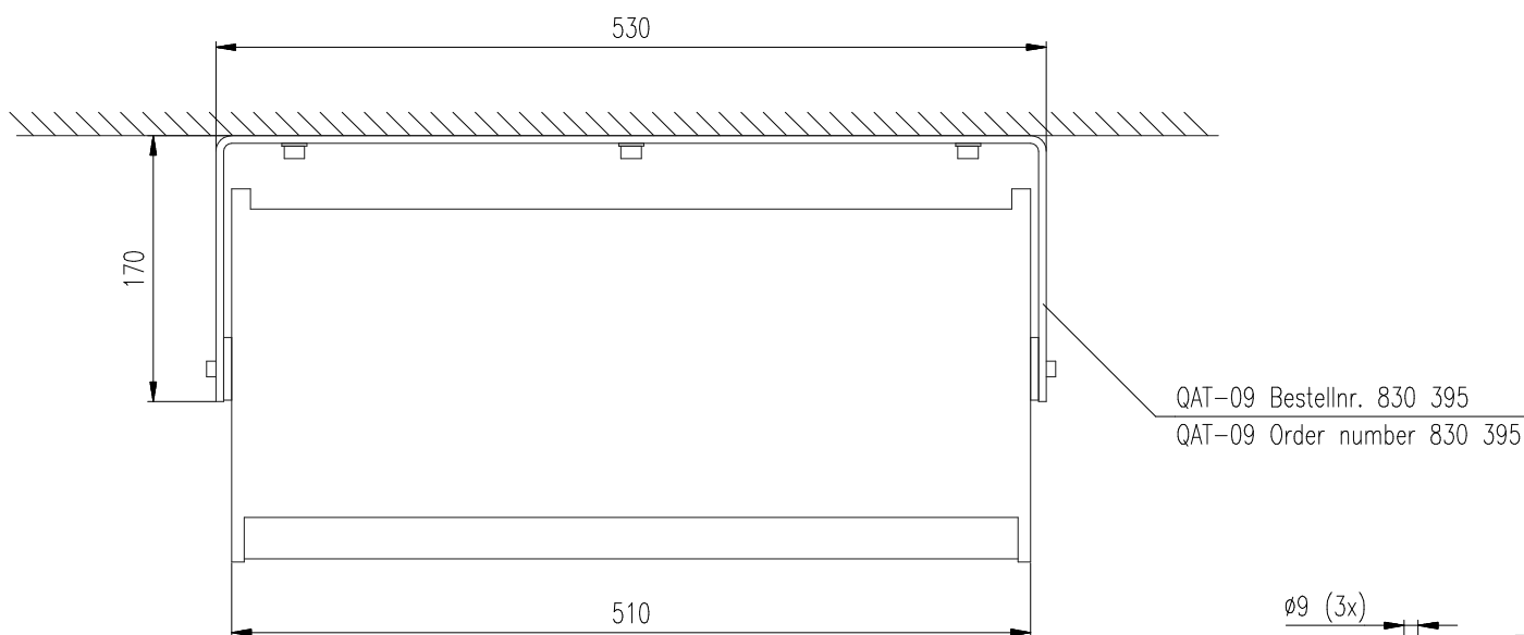
Ansicht von oben / Top view
