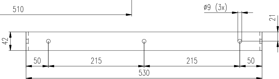
Ansicht von oben / Top view
